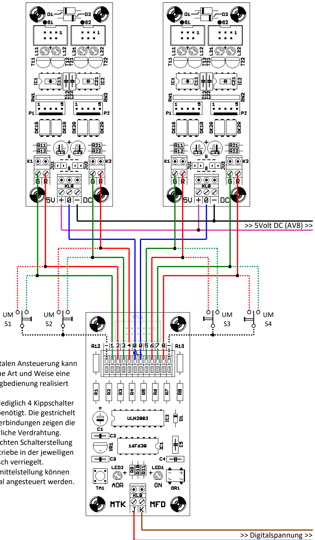
Anschluss- / Verdrahtungsplan MFD < > SC2
